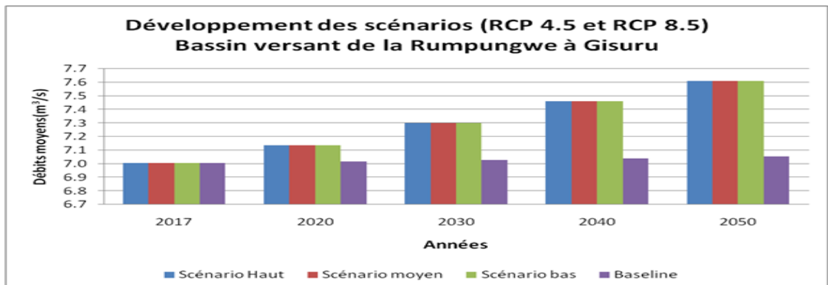
Figure 22: Développement des scénarios des débits moyens des ressources en eau
