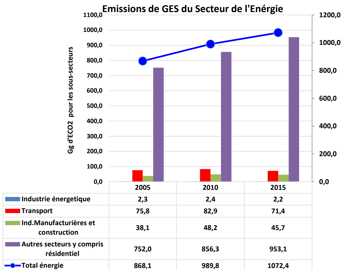
Figure 8: Tendances des émissions pour le secteur de l'énergie
